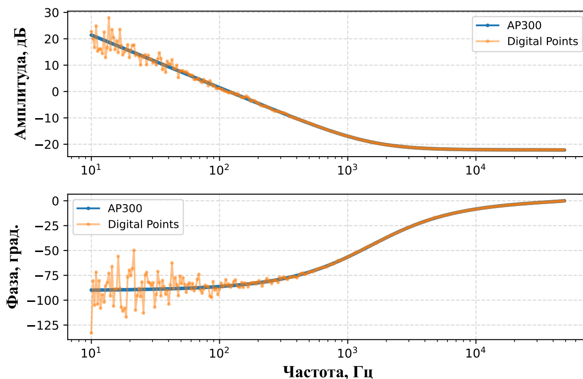
Рисунок А.1 – Измеренные частотные характеристики
