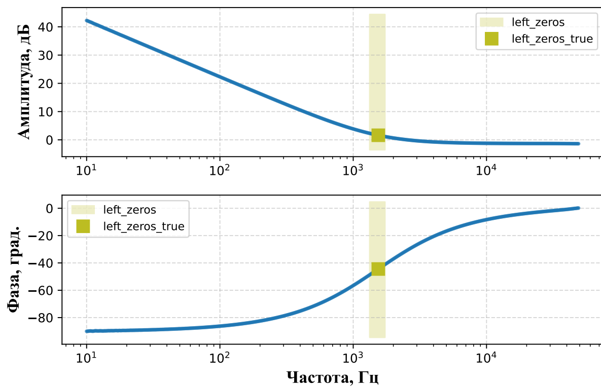
Рисунок А.2 – Частотные характеристики ПИ-регулятора контура регулирования тока (внутрисхемное измерение)
