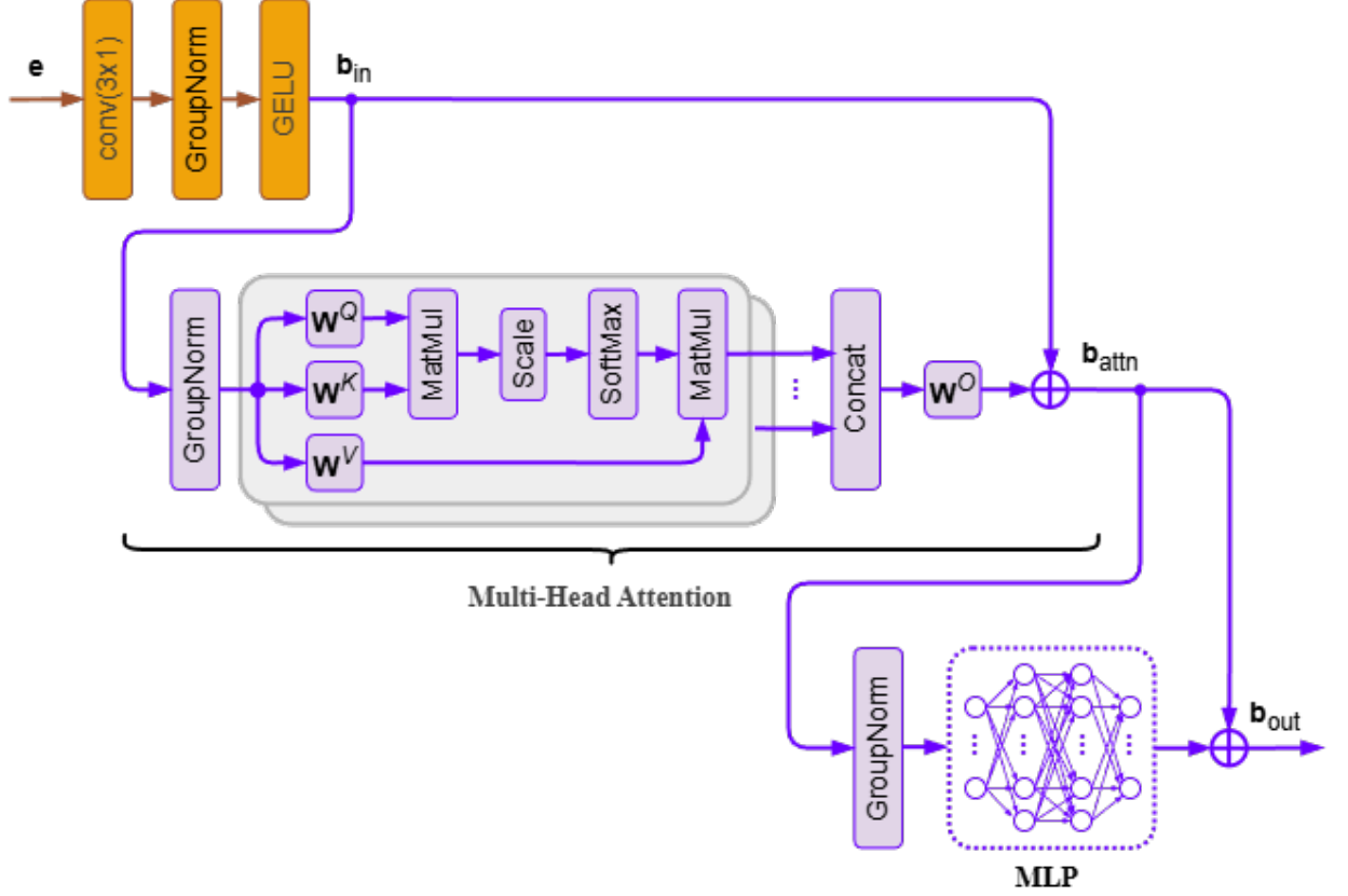
Рисунок 3.3. Блок-схема bottleneck-алгоритма
