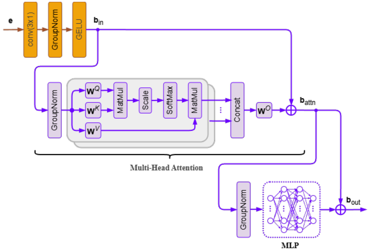
Рисунок 3.3. Блок-схема bottleneck-алгоритма
