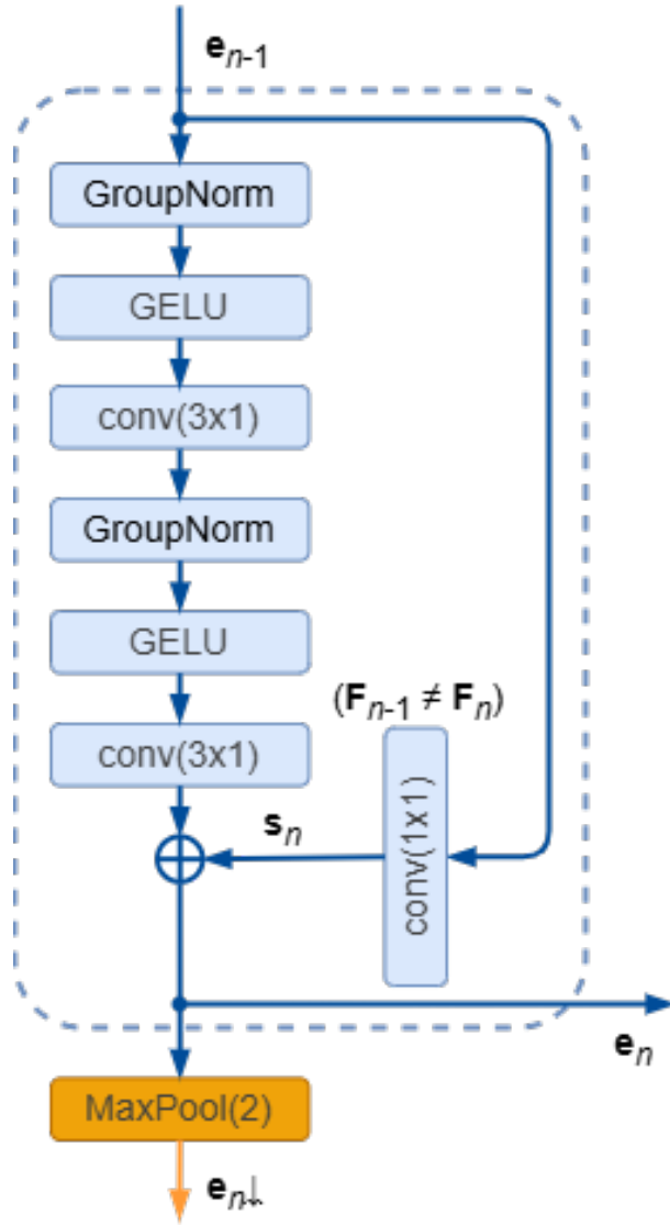
Рисунок 3.2. Блок-схема базового блока энкодера
