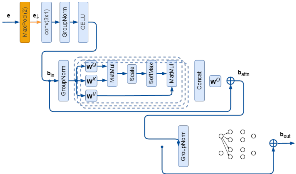
Рисунок 3.3. Блок-схема bottleneck-алгоритма
