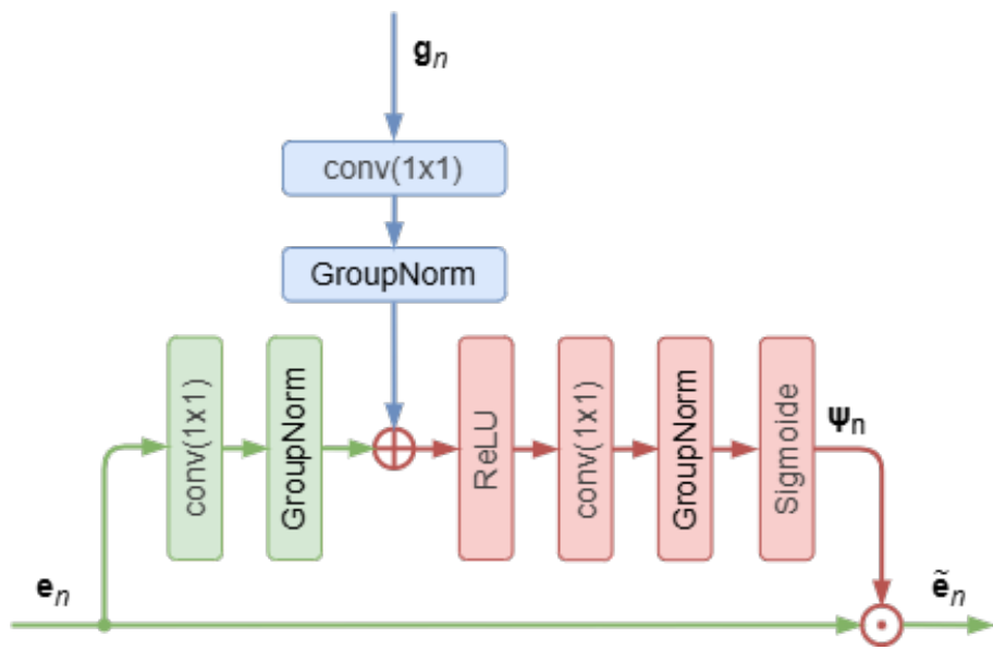
Рисунок 3.4. Блок-схема «взвешивания» обходных связей
