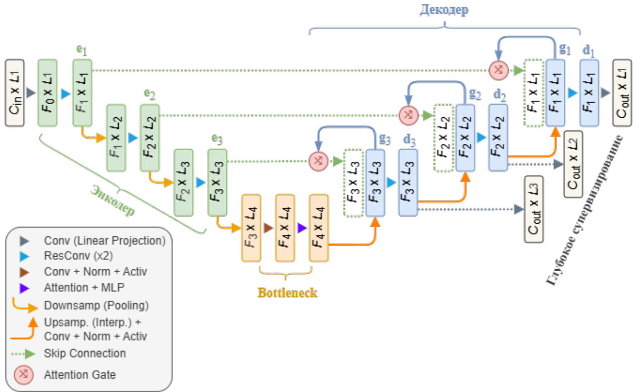
Рисунок 3.1. Блок-схема архитектуры модели
