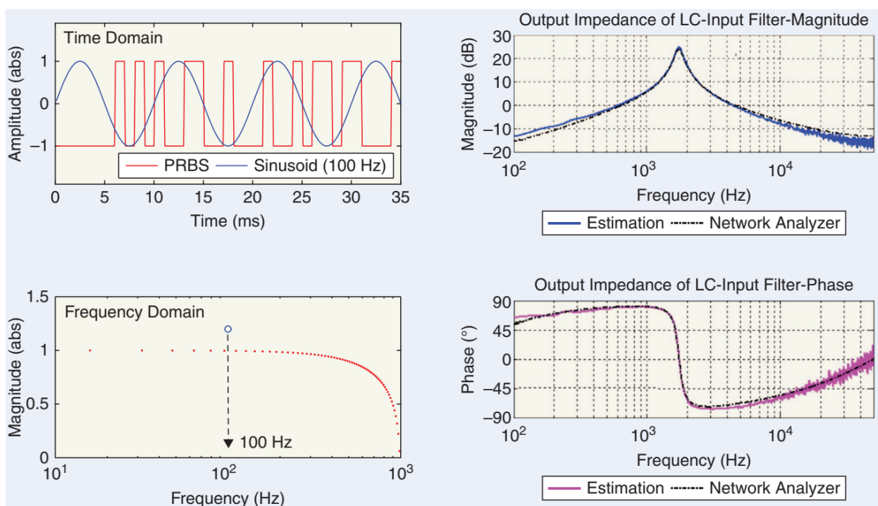
Рисунок 1.1. Алгоритм PRBS
