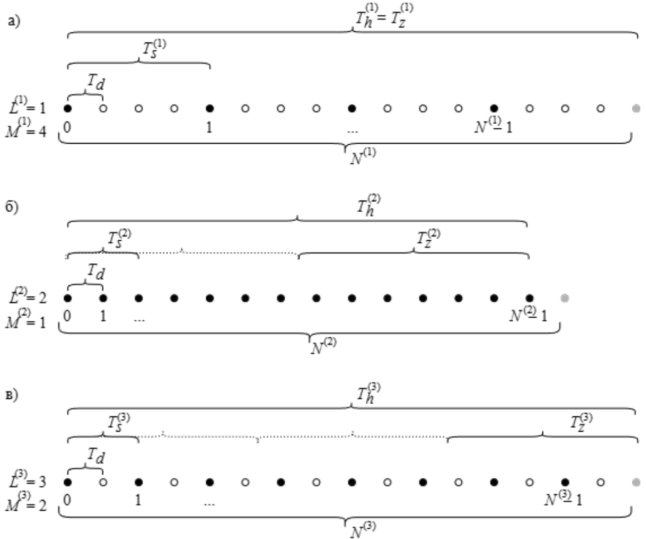
Рисунок 2.5. Параметры N, M, L алгоритма при T_z^{(k)} = var
