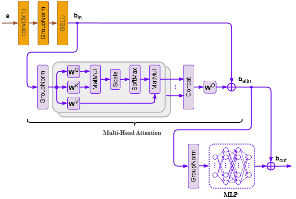
Рисунок 3.3. Блок-схема bottleneck-алгоритма
