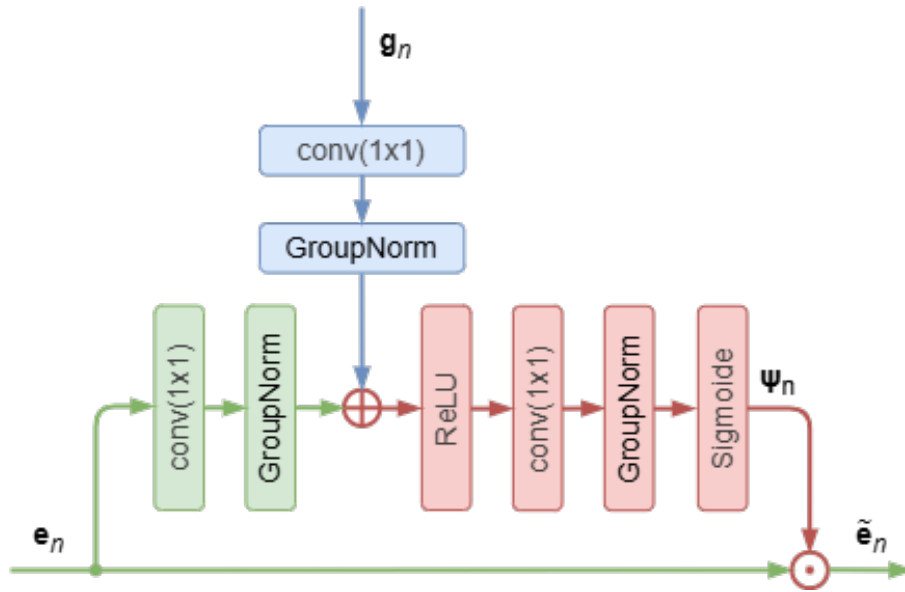
Рисунок 3.4. Блок-схема «взвешенных» обходных связей энкодера с декодером
