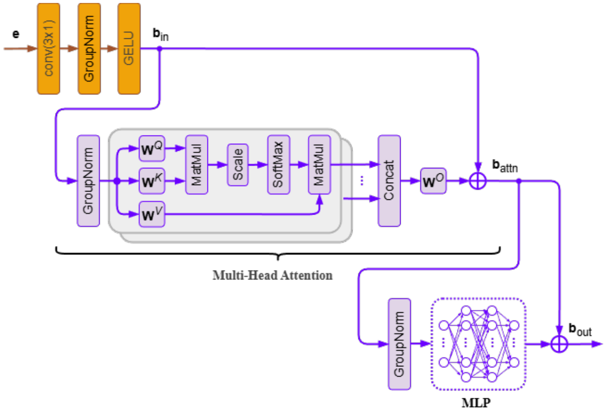
Рисунок 3.3. Блок-схема bottleneck-алгоритма
