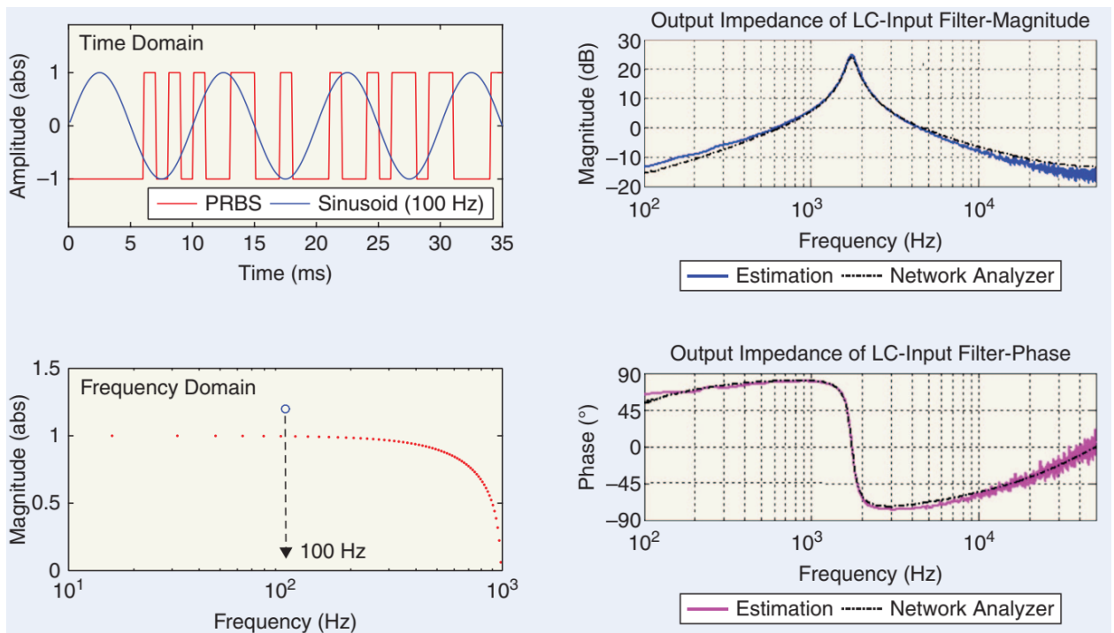
Рисунок 1.1. Алгоритм PRBS
