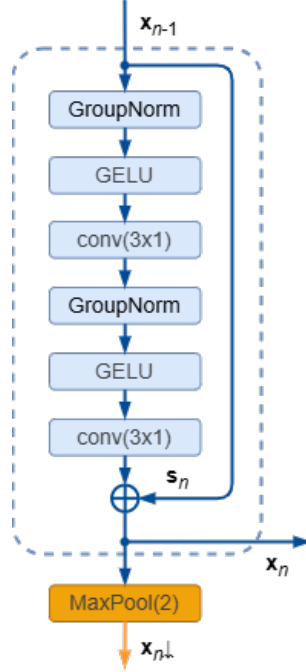
Рисунок 3.2. Блок-схема базового блока энкодера
