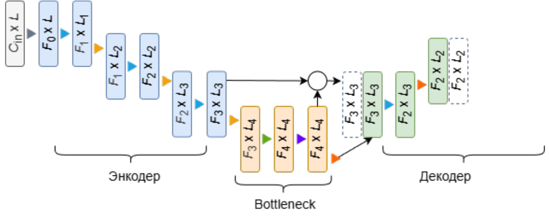
Рисунок 3.1. Блок-схема архитектуры модели
