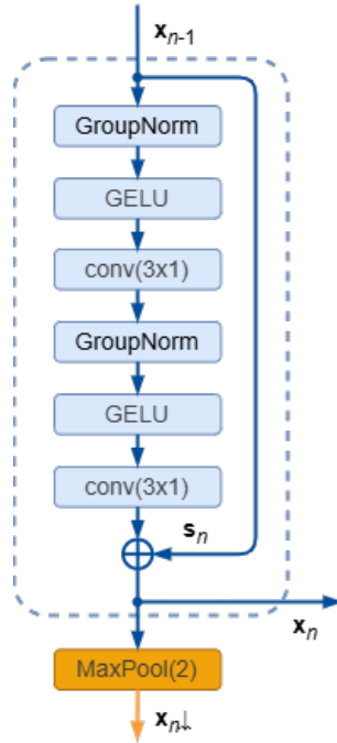
Рисунок 3.3. Блок-схема bottleneck-алгоритма
