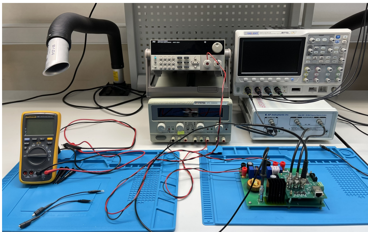
Рисунок А.1. Лабораторный стенд
