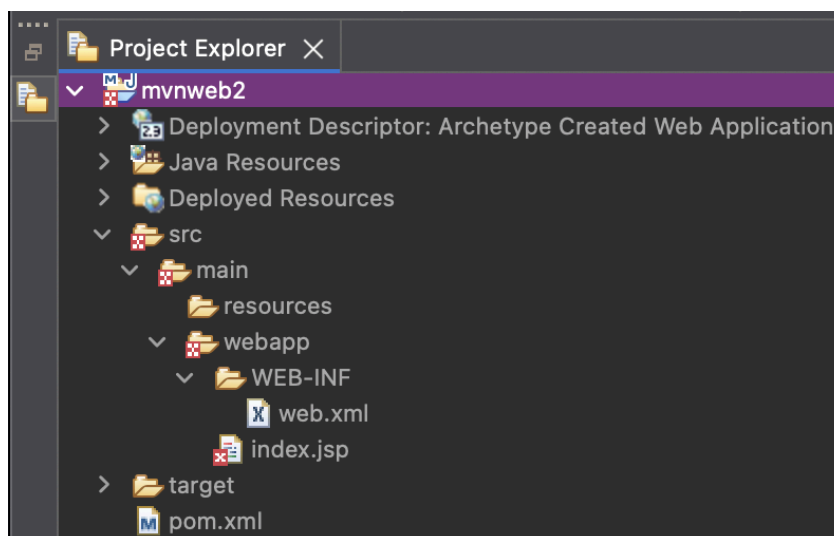
Рис. 1 – Структура созданного Maven-проекта
