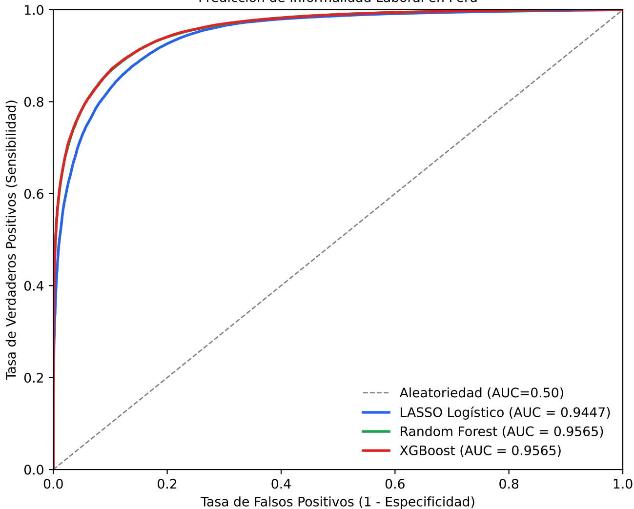
Figura: Curvas ROC — Comparación de Modelos Predicción de Informalidad Laboral en Perú
