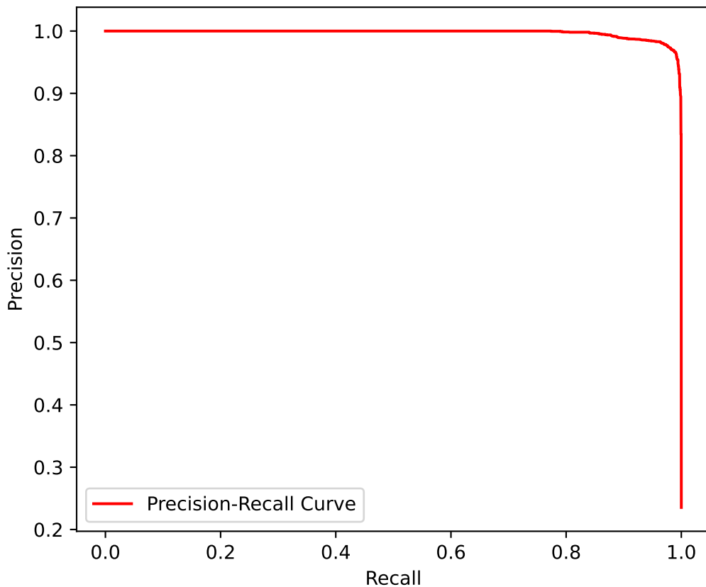
Precision-Recall Curve - Classe 2
