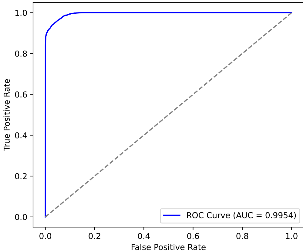
ROC Curve - Classe 0
