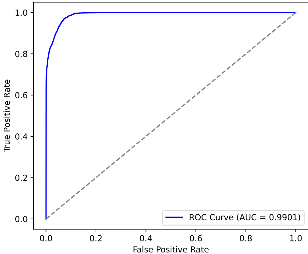
ROC Curve - Classe 1
