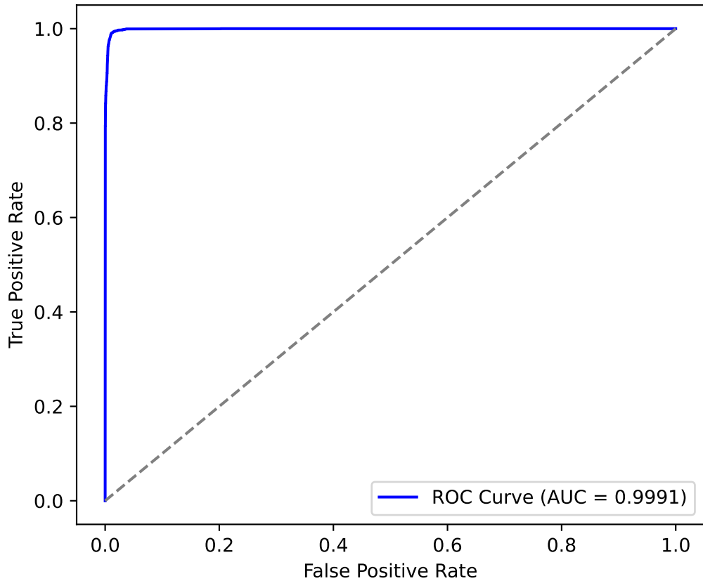
ROC Curve - Classe 2
