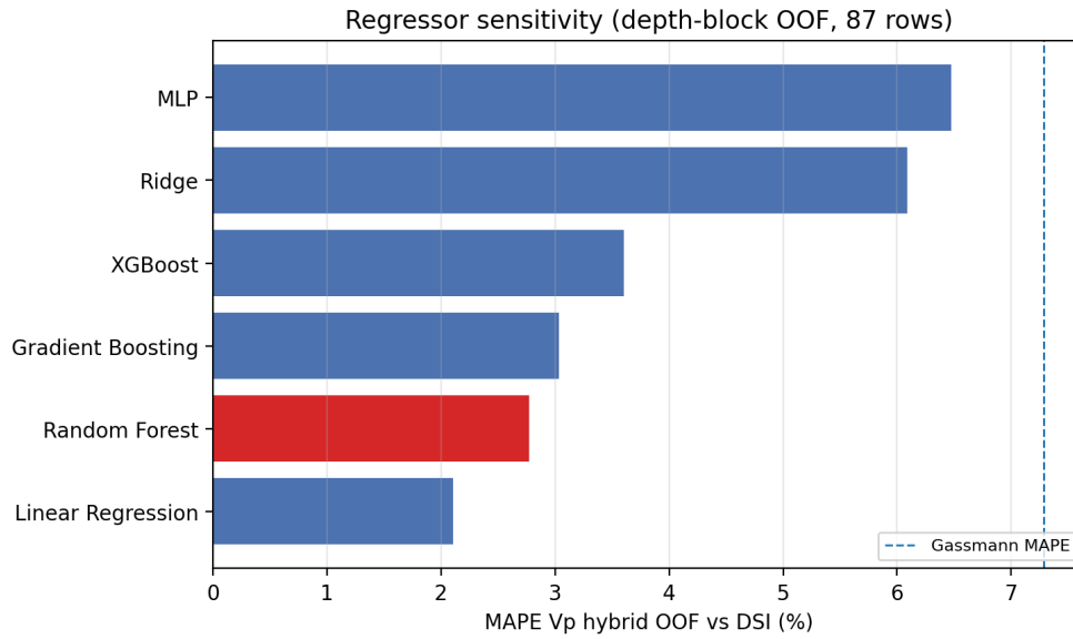
Figura 2: MAPE de V_p híbrida OOF versus DSI por regressor. Linha tracejada: baseline Gassmann (7,3%). Todos os seis regressores ficam abaixo do baseline; RF (barra vermelha) permanece o modelo adotado e a regressão linear apresenta o menor MAPE nesta rodada.
