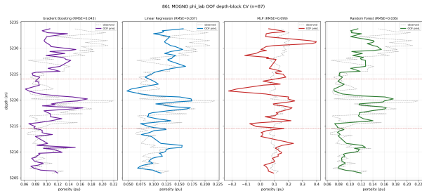
Observado (tracejado) versus OOF (colorido) por regressor
