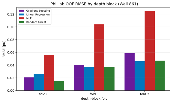
RMSE OOF por bloco: RF, GB, MLP e LR ( \phi_{lab} )
