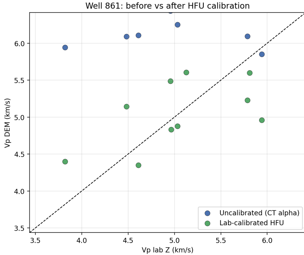
Figura 3: V_p antes e depois da calibração por HFU nos plugs de laboratório. Após o ajuste, os pontos aproximam-se da linha 1:1.
