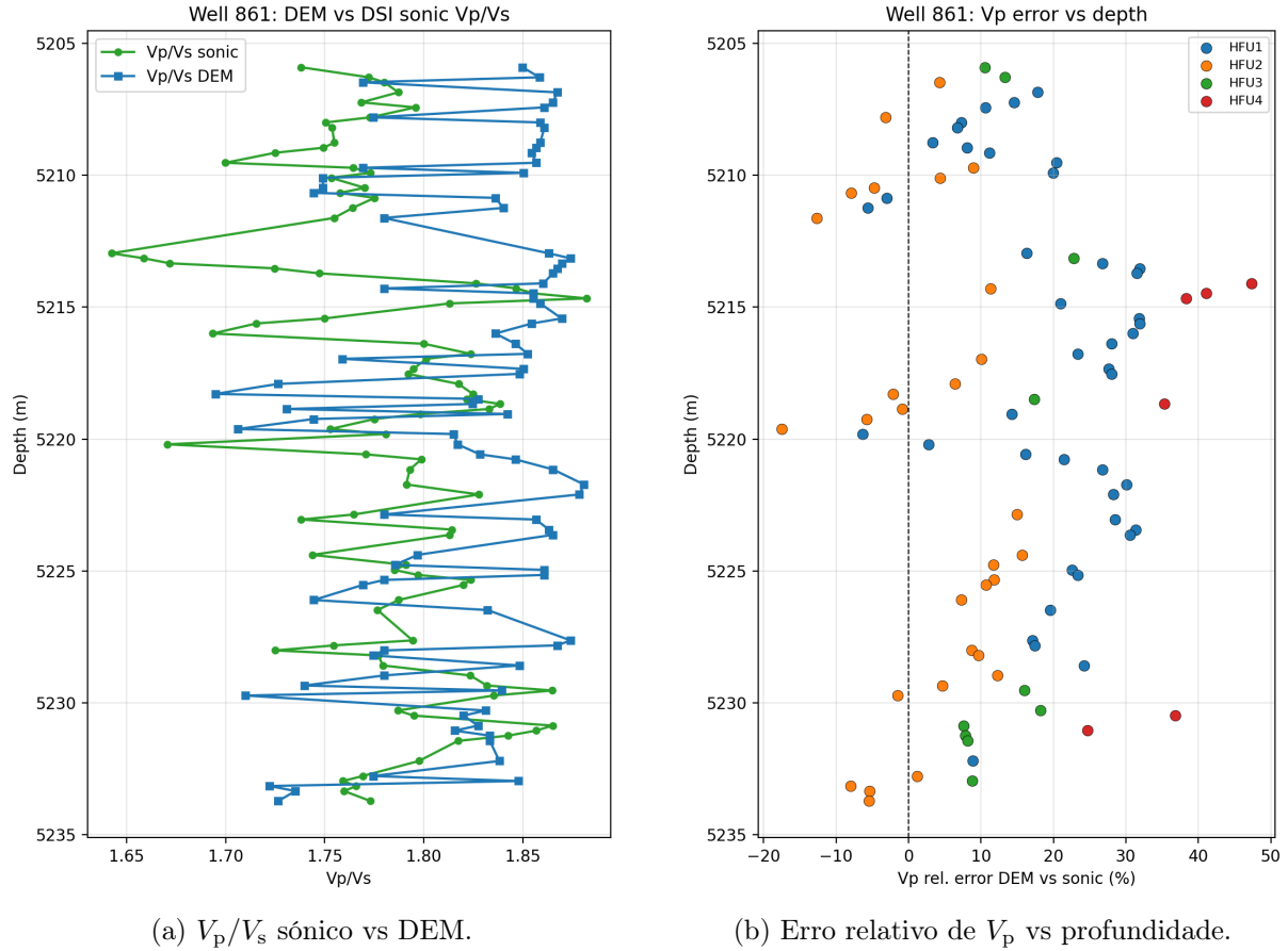
Figura 9: Valida33o complementar: raz33o V_p/V_s e erro percentual.
