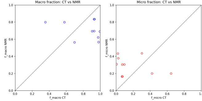
Figura 11: Frações macro CT versus NMR nos dez plugs com microCT. A correlação é fraca ( r \approx -0,30 ), alertando para não tratar CMFF/BFV como proxy direto da segmentação CT.
