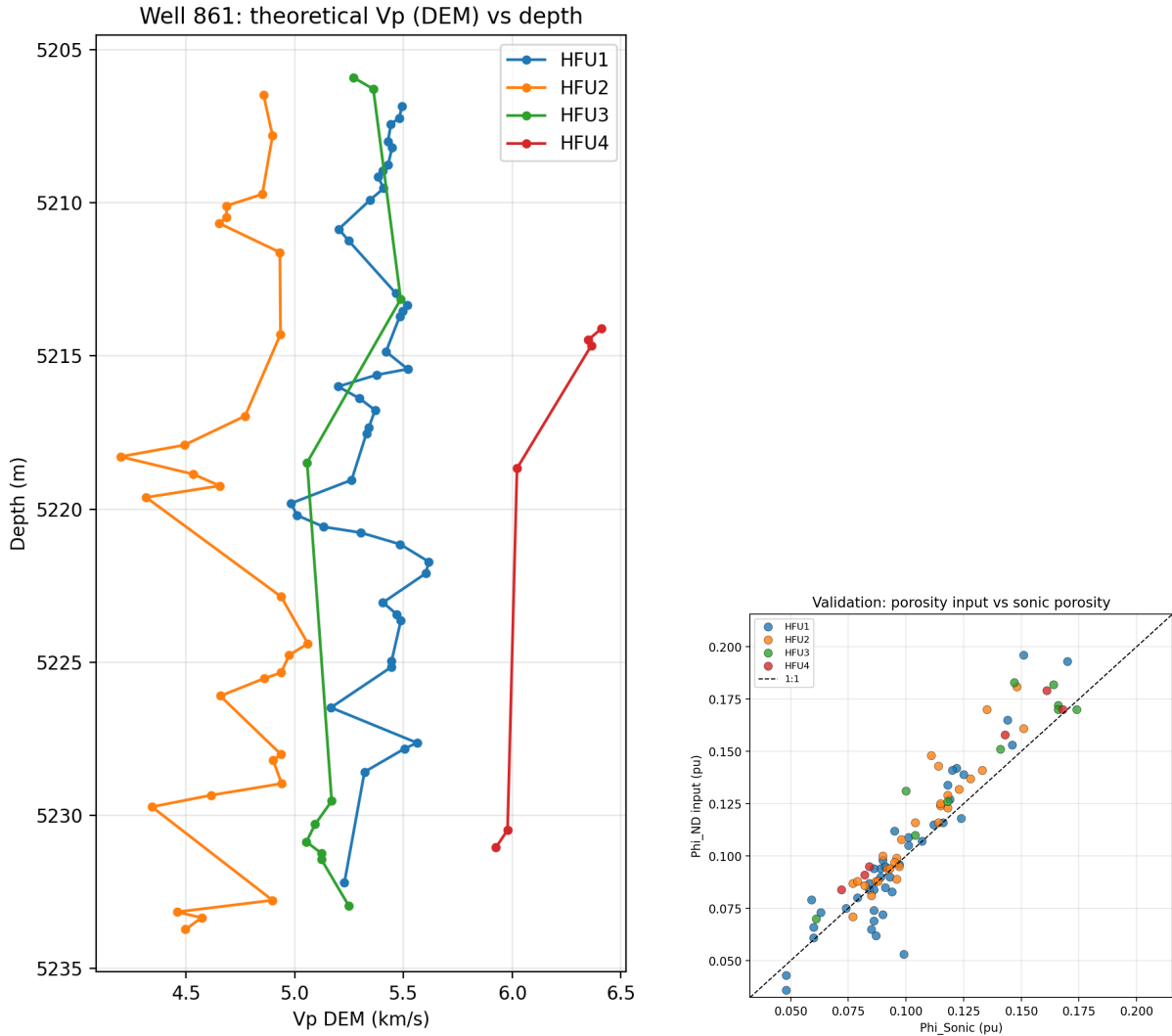
(a) V_p DEM versus profundidade por HFU.
