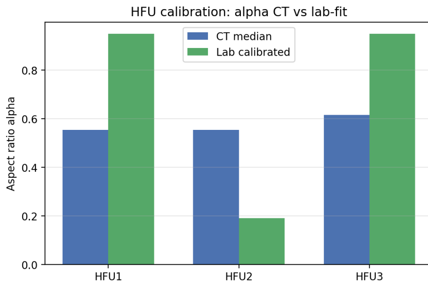
Figura 4: Razão de aspecto calibrada versus mediana do microCT por HFU. Barras divergentes indicam que a geometria CT, sozinha, não fecha o laboratório.
