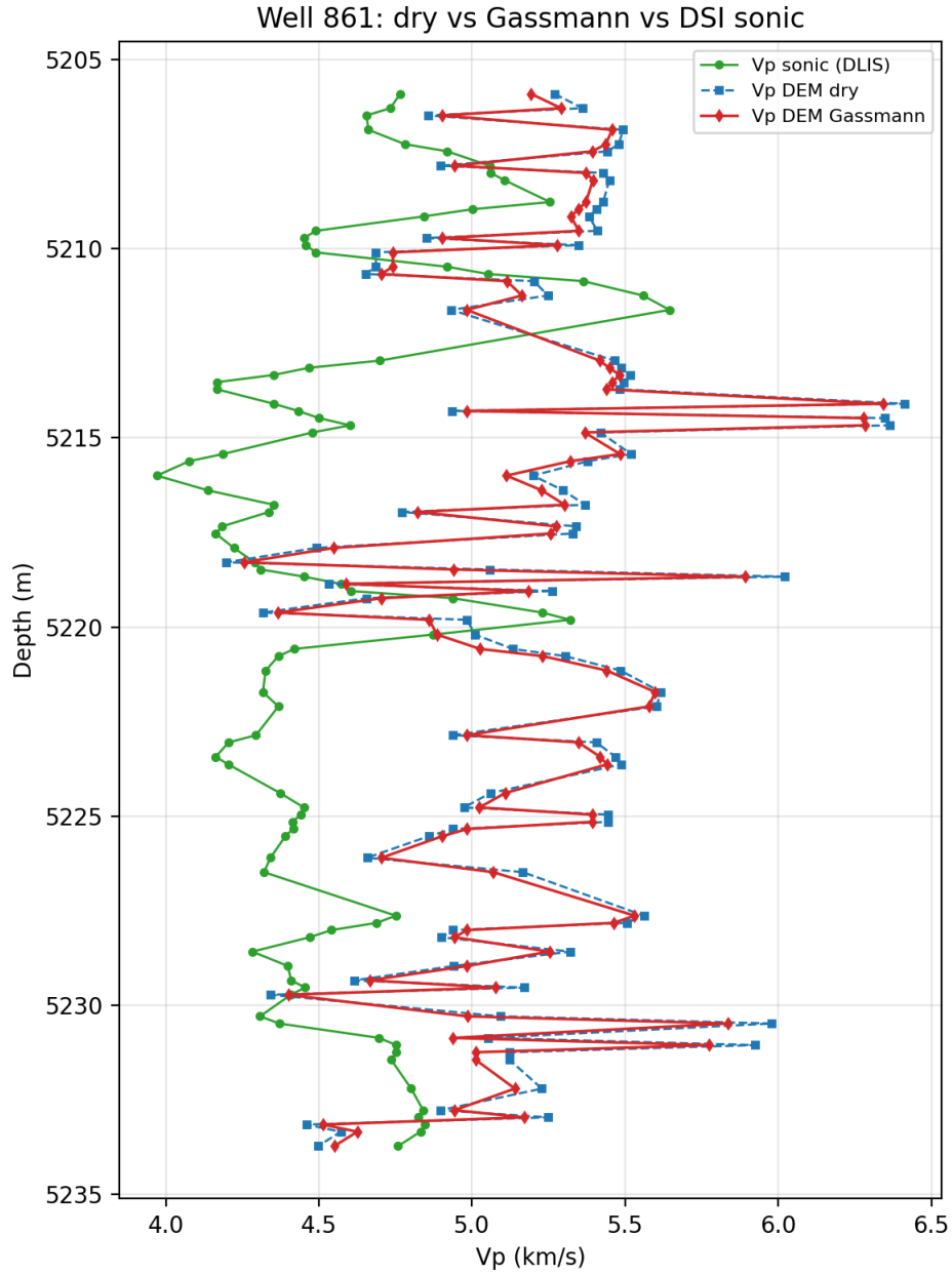
Figura 10: Trilha de profundidade: V_p sônico (verde), DEM seco (azul tracejado) e DEM com Gassmann (vermelho). A saturacao aproxima parcialmente o sônico, mas não elimina o viés sistemático.
