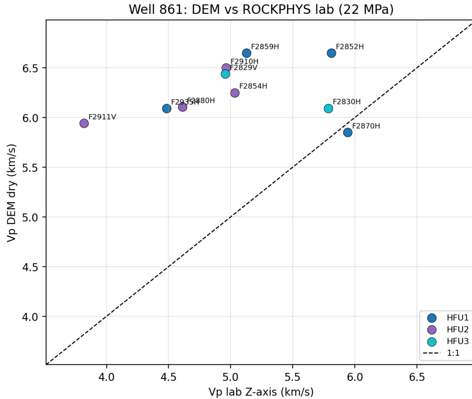
Figura 2: V_p DEM versus V_p de laboratório (eixo Z , 22,1 MPa), antes da calibração por HFU. Pontos acima da diagonal indicam superestimação do modelo.
