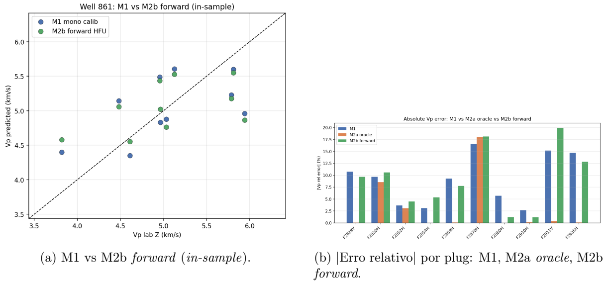
Figura 5: Teste A/B multiescala (fase 2f): o modo forward nao supera o monoescala calibrado de forma consistente.
