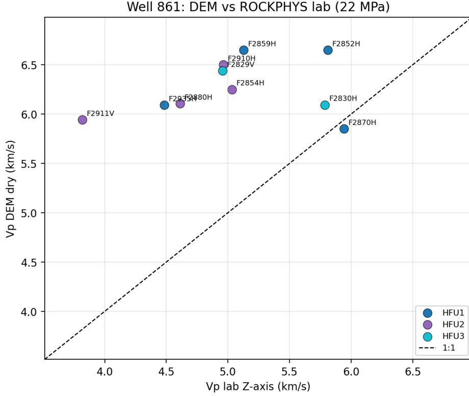
Figura 5: V_p DEM versus V_p de laboratório (eixo Z , 22,1 MPa), antes da calibração por HFU. Pontos acima da diagonal indicam superestimação do modelo.
