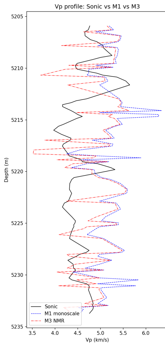
(b) Trilha de V_p : sónico, M1 e M3.
