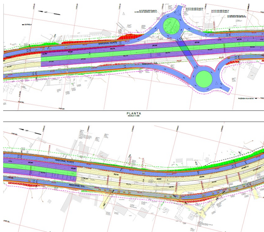
Figura 2 - Proposta de dispositivo em desnível encaminhada pela concessionária.
