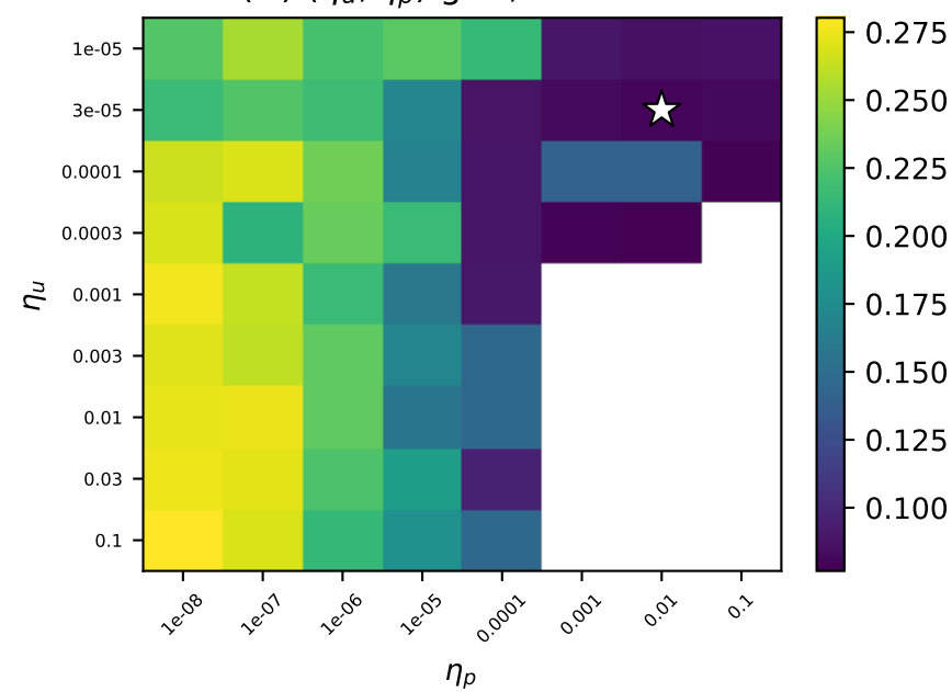
(D) (\eta_u, \eta_p) grid, \lambda = 1000
