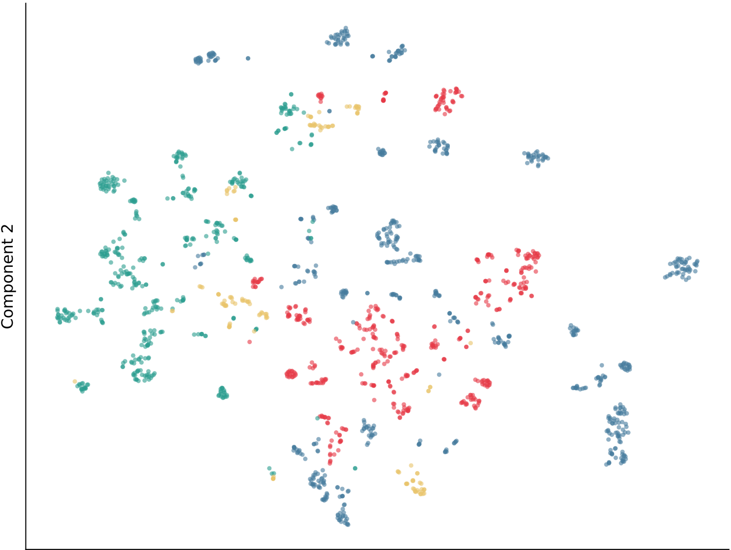
t-SNE
