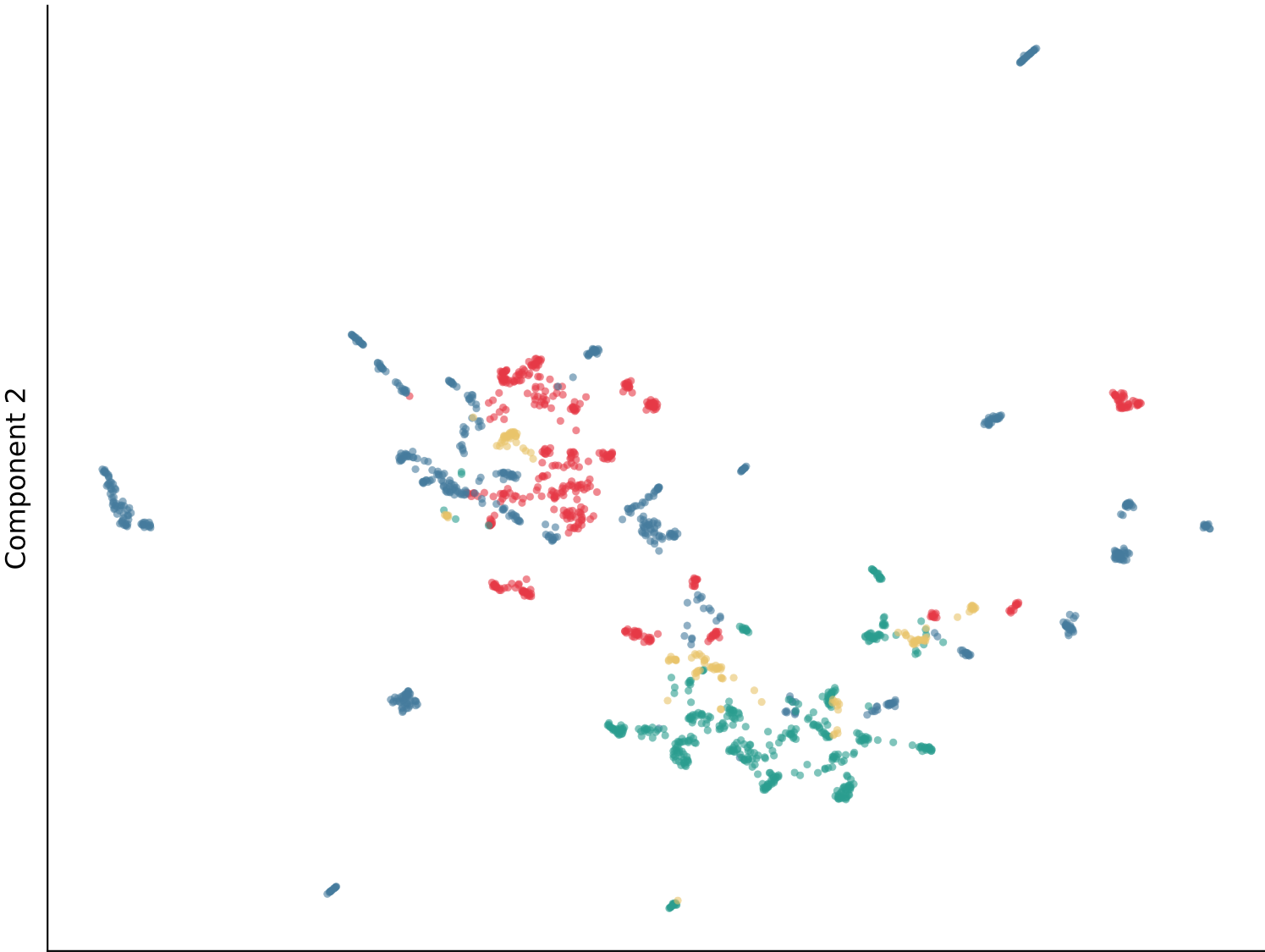
UMAP
