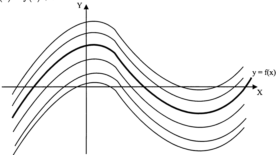
Fig. 11.3 - Linhas de nível da função \varphi(x, y) = y - f(x) .
