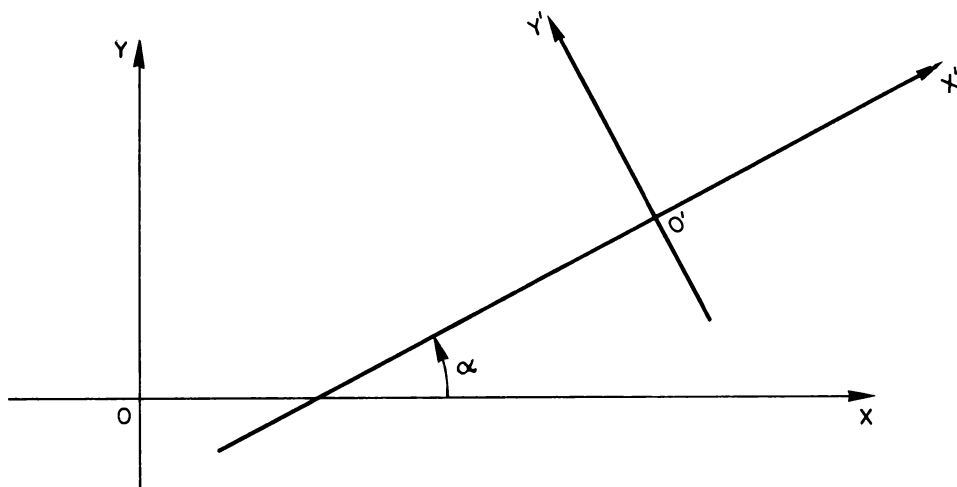
Fig. 23.6 - O ângulo \alpha entre os eixos OX e O'X' .
