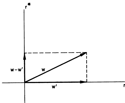
Fig. 21.1 - A projeção ortogonal w' do vetor w sobre a reta r .
