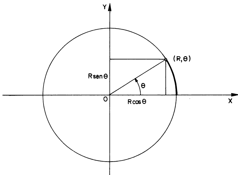
Fig. 3.4 - Sistema de coordenadas polares.
