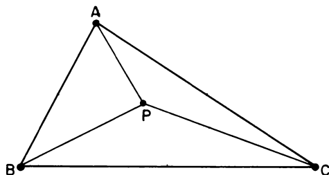
Fig. 36.1 - As coordenadas baricêntricas do ponto P obtêm-se a partir das áreas dos triângulos APC , ABP , BCP e ABC .
