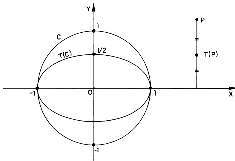
Fig. 24.1 - Uma compressão vertical do plano.
