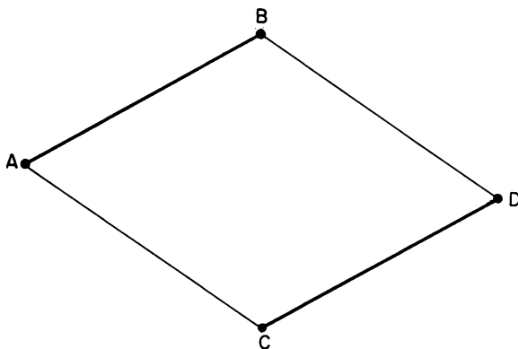
Fig. 18.1 - Segmentos orientados equipolentes.
