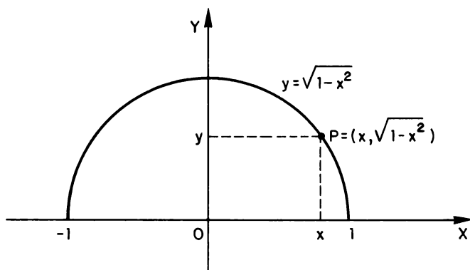
Fig. 5.1 - A semi-circunferência y = \sqrt{1-x^2} , -1 \leq x \leq 1 .
