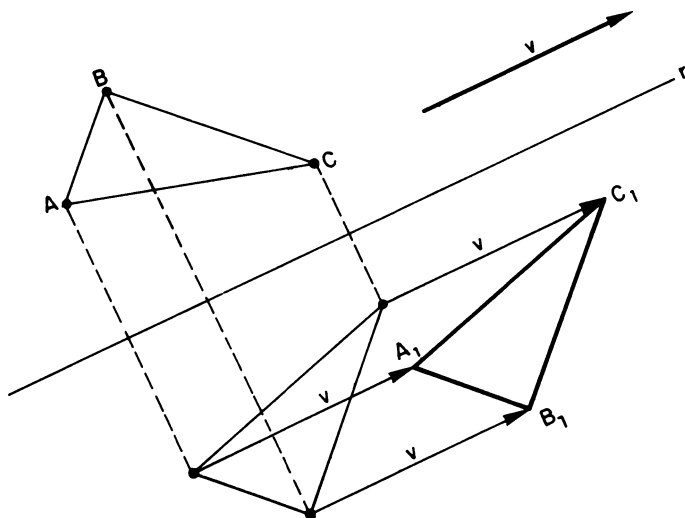
Fig. 27.4 - O triângulo A_1, B_1, C_1 , imagem do triângulo ABC pela reflexão em torno de r com vetor de deslizamento v .
