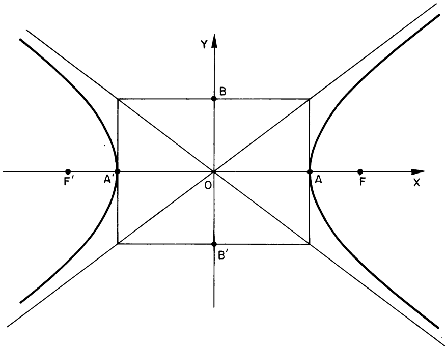
Fig. 4.6 - Hipérbole de equação \frac{x^2}{a^2} - \frac{y^2}{b^2} = 1 .
