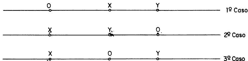
Fig. 2.2 - Provando que d(X, Y) = |x - y| .
