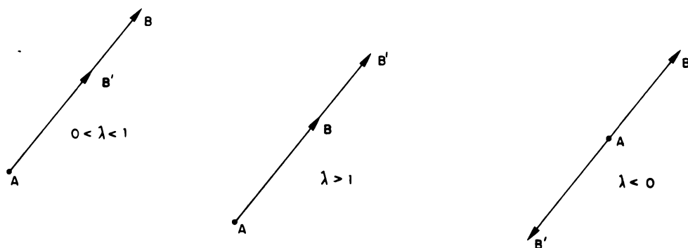
Fig. 18.5 - \overrightarrow{AB'} = \lambda \cdot \overrightarrow{AB} em três casos, para diferentes valores de \lambda .
