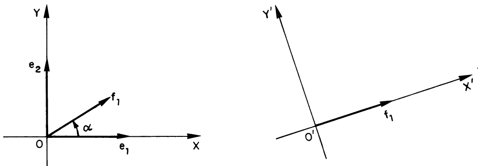
Fig. 23.1 - O ângulo \alpha , entre os vetores e_1 e f_1 .
