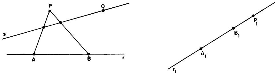
Fig. 38.1 - Uma colinação que levasse os três vértices de um triângulo em três pontos não colineares não seria sobrejetiva.
