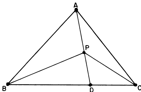
Fig. 36.2 - Se P = \alpha \cdot A + \beta \cdot B + \gamma \cdot C então \alpha = d(P, D)/d(A, D) .
