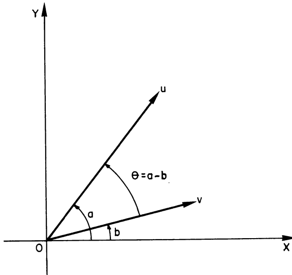
Fig. 19.3 - Usando vetores em Trigonometria.
