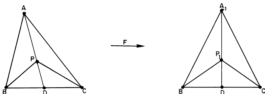
Fig. 36.4 - A transformação afim F deixa fixos B , D e C e leva A em A_1 de modo que A_1D seja a altura de A_1BC .
