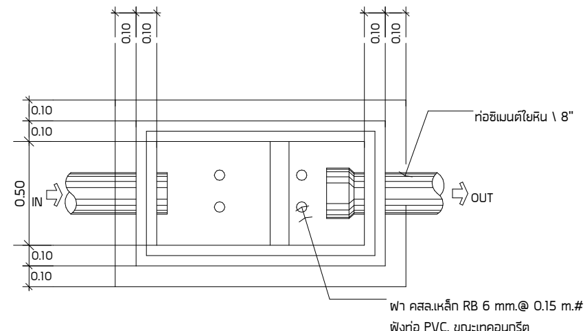
แปลนขยายบ่อดักขยะ-ไขมัน Scale 1:25
