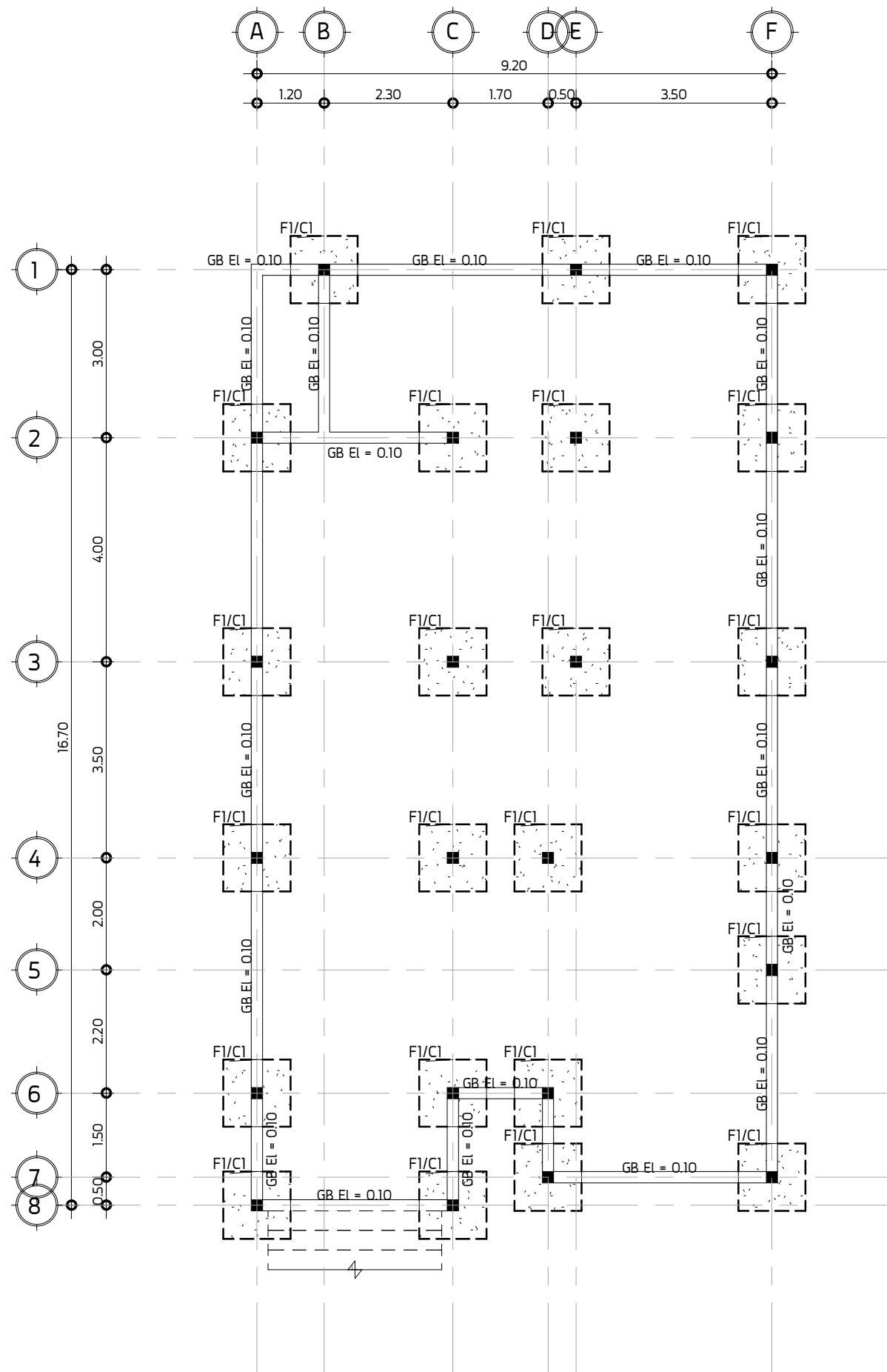
แปลนฐานราก มาตราส่วน 1 : 100
