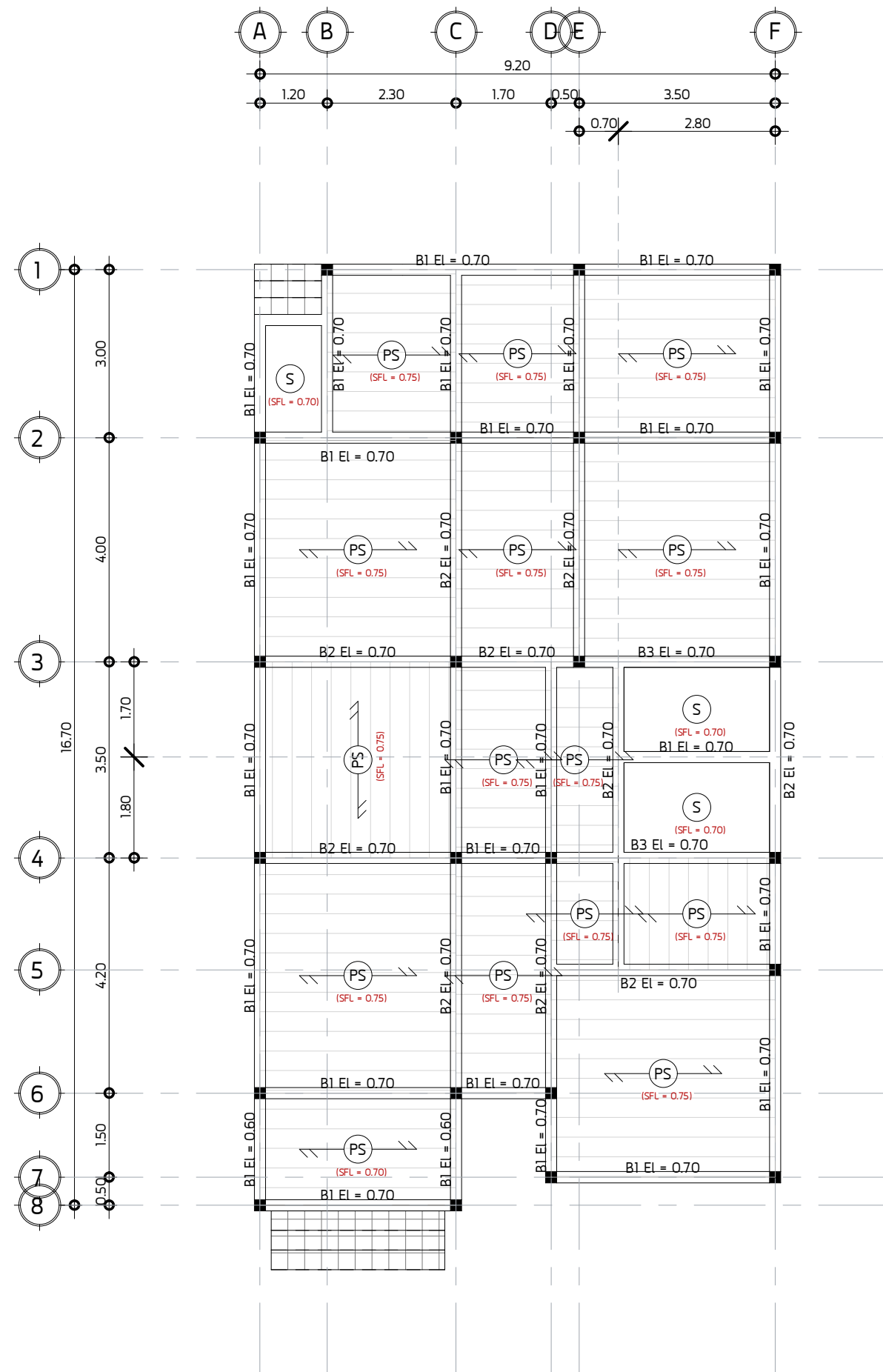
แปลนคานพื้น มาตราส่วน 1 : 100
