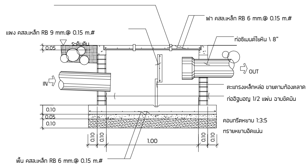
รูปตัดขยายบ่อตกขยะ-ไขมัน Scale 1:25
