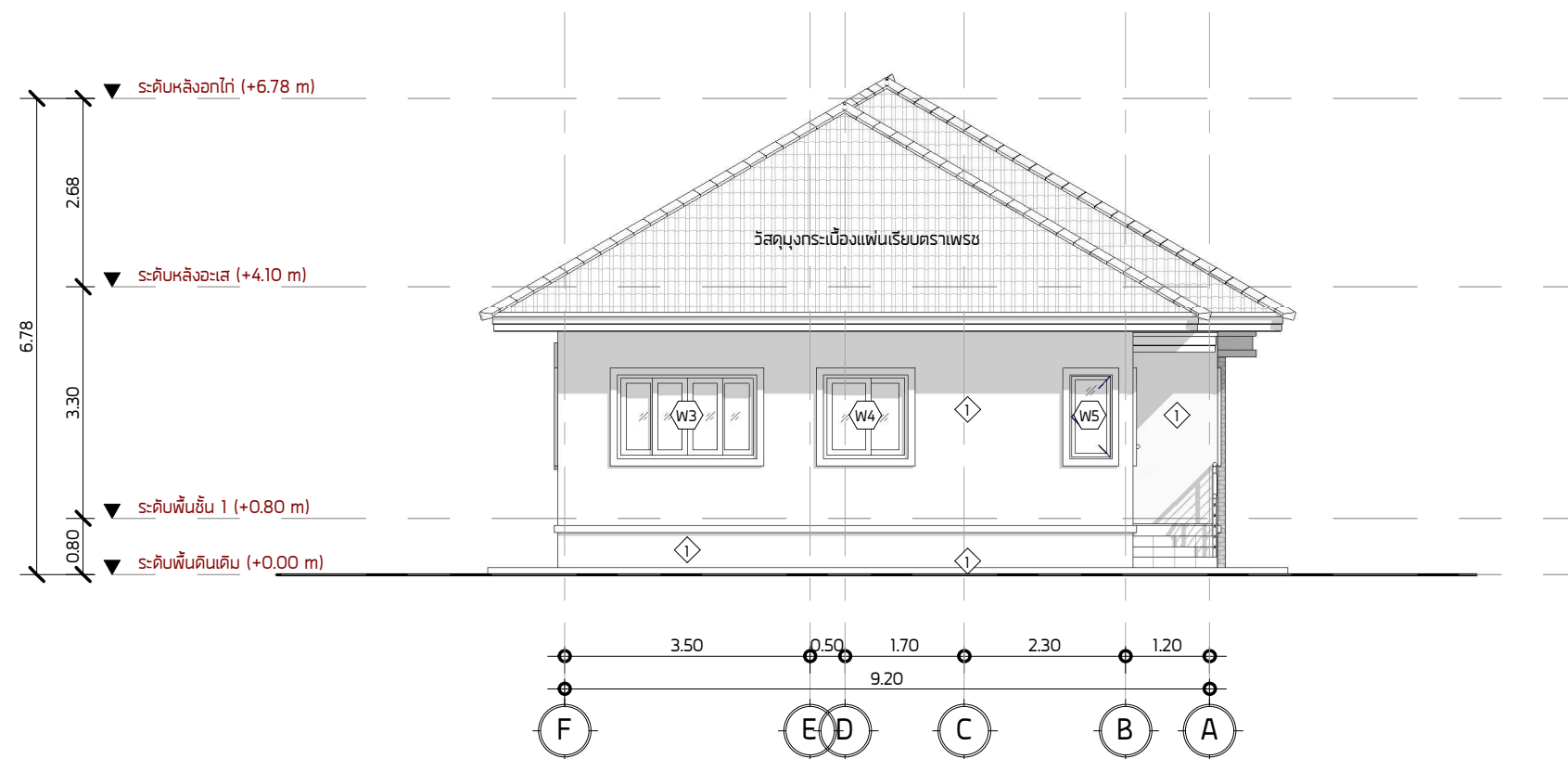
รูปด้าน 3 SCALE : 1 : 100
