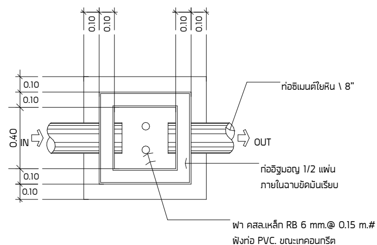
แปลนขยายบ่อพักน้ำทิ้ง (HH) Scale 1:25
