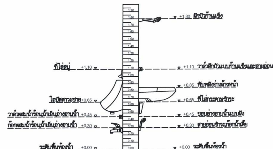
แบบขยายการจัดตั้งอุปกรณ์ห้องน้ำ
