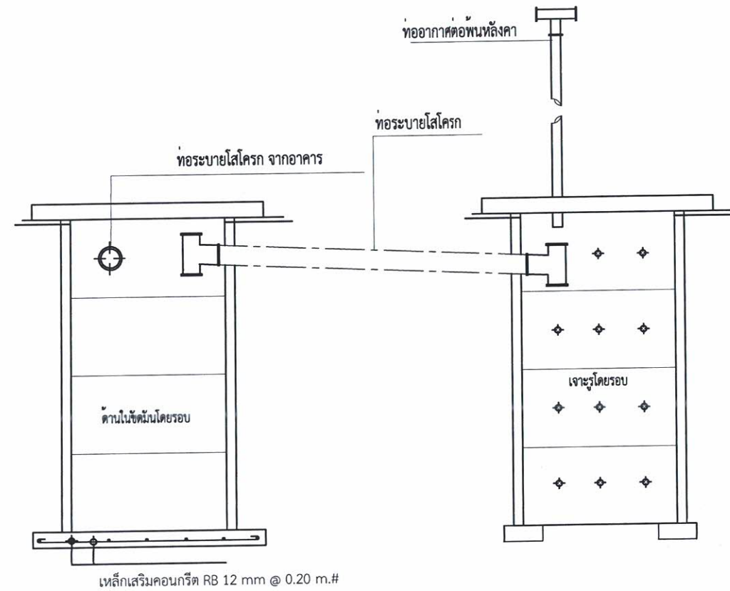
รูปตัดบ่อเกรอะ - บ่อซึม
