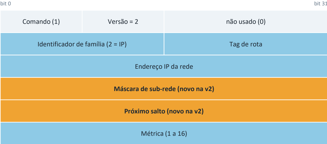
Cabeçalho de 4 bytes + até 25 entradas de 20 bytes (504 bytes por mensagem)
