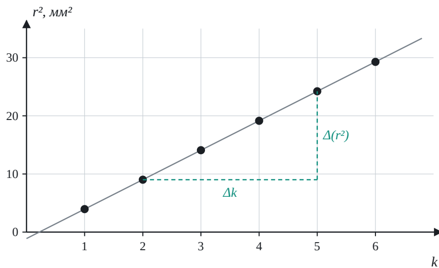
Рис. 14. Примерный вид зависимости r_k^2 от номера кольца
