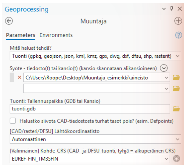
Kuva 5. Tuonti: syötteenä kansio, tallennuspaikkana tuonti.gdb. CAD-asetukset näkyvät, koska kansiossa on DWG/DXF-tiedostoja.
