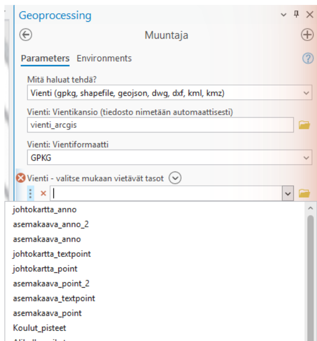
Kuva 9. Tasot valitaan aktiivisen kartan tasoista pudotusvalikosta.
