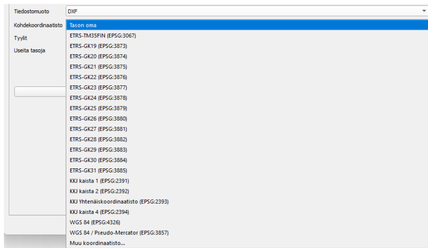
Kuva 11. Kohdekoordinaatistot: ETRS-TM35FIN, ETRS-GK19–GK31, KKI-kaistat, WGS 84, Web Mercator ja muu koordinaatisto.
