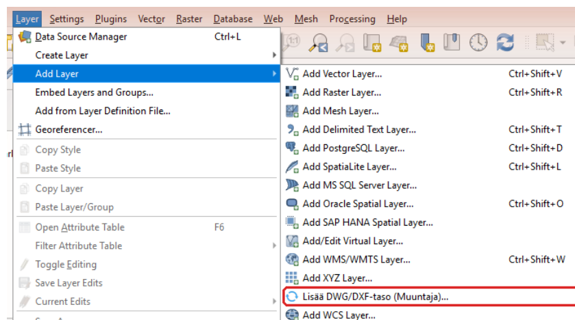
Kuva 9. DWG/DXF-tason lisääminen Layer-valikosta.
