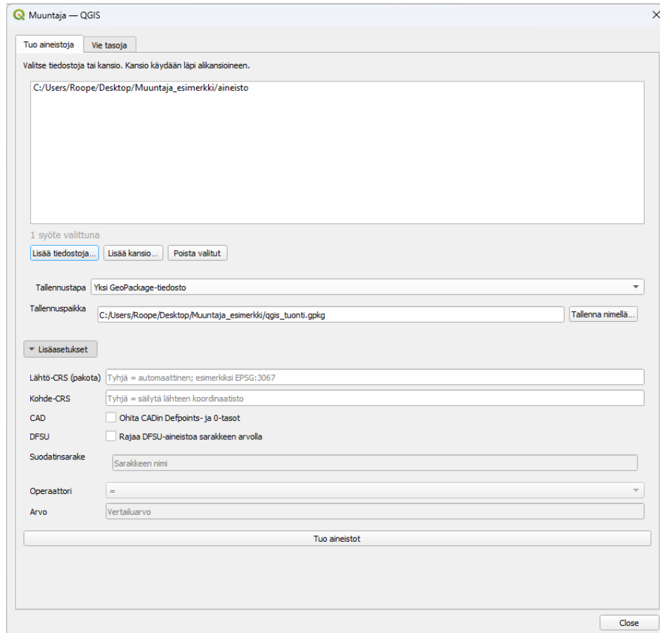
Kuva 6. Tuonti: syötteenä kansio, tulos yhteen GeoPackageen. Lisäasetukset avattuna.
