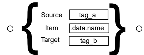
Extract JSON
