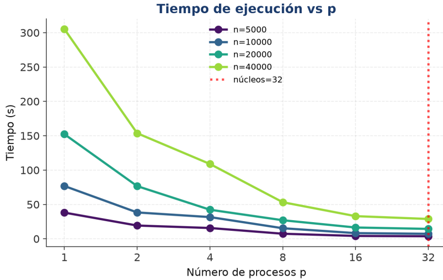
Figura 1: Tiempo vs p (Khipu, 32 núcleos). La reducción T_{\text{reduce}} es \leq 3,6\% (y < 1\% para n grande): el cuello no es la comunicación.
