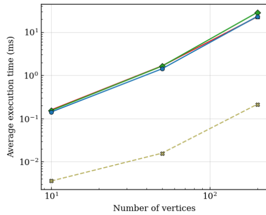
(b) Classe graphe.
