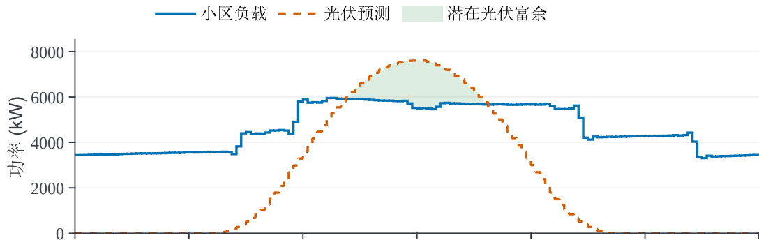
(a) 日内负载与光伏供需关系
