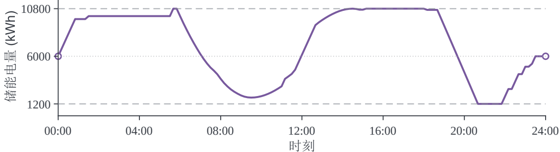
(c) 储能电量与运行边界
