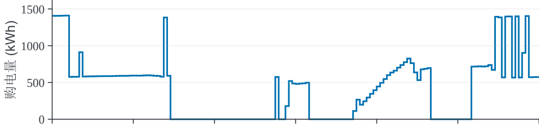
(a) 最优计划购电量
