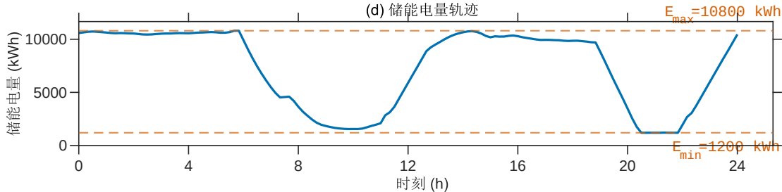
(d) 储能电量轨迹
