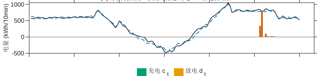
(c) 储能日内充放电动作 (must/max 尽限规则)
