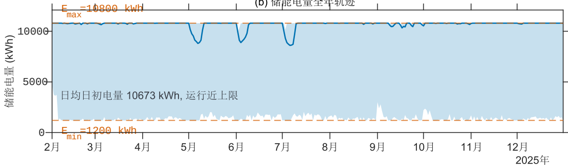
(b) 储能电量全年轨迹
