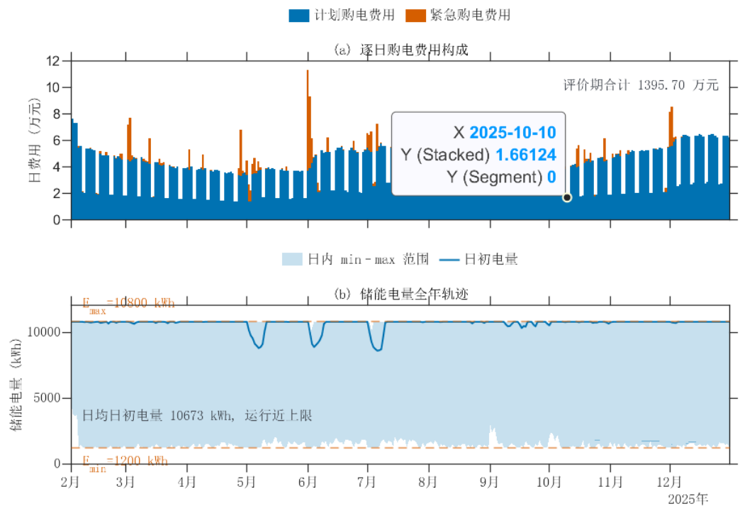
图 8 逐日购电费用构成与储能电量全年轨迹
