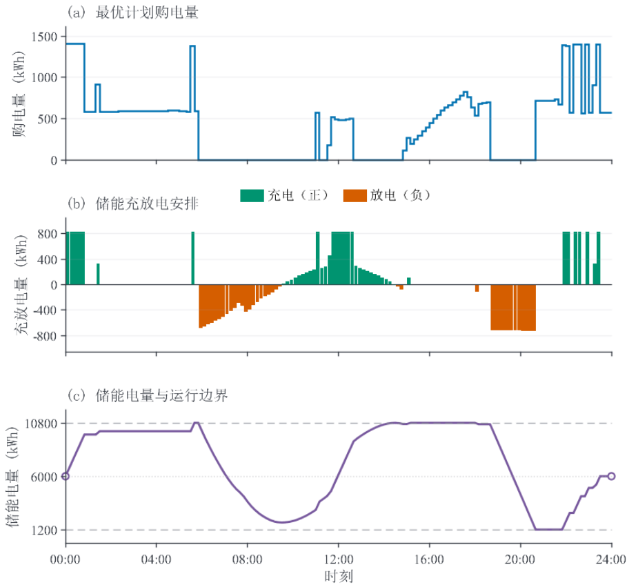
图 3 最优购电与储能运行策略：计划购电量、储能充放电动作与储电量轨迹
