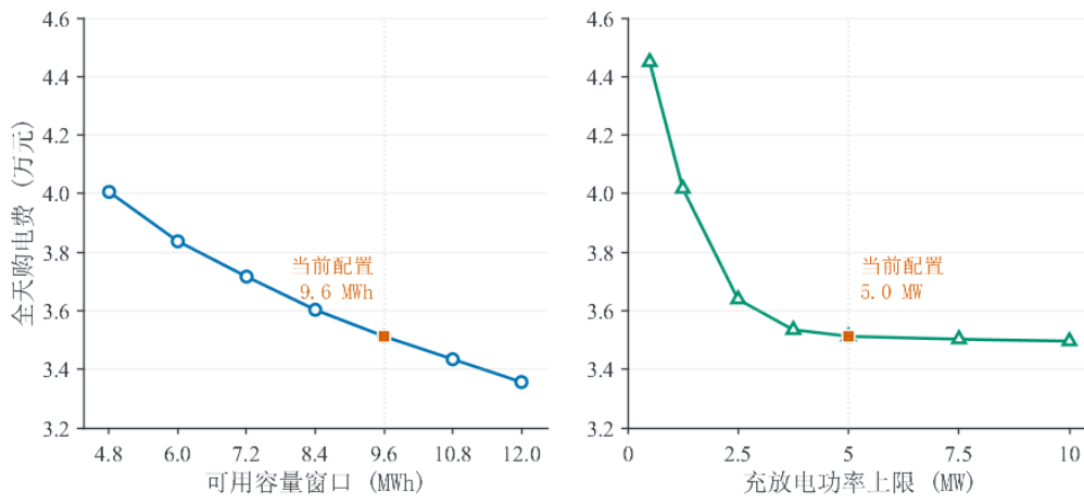
图 4 容量窗口与功率上限的敏感性（保持 E_0 = E_{144} = 6000 kWh）
