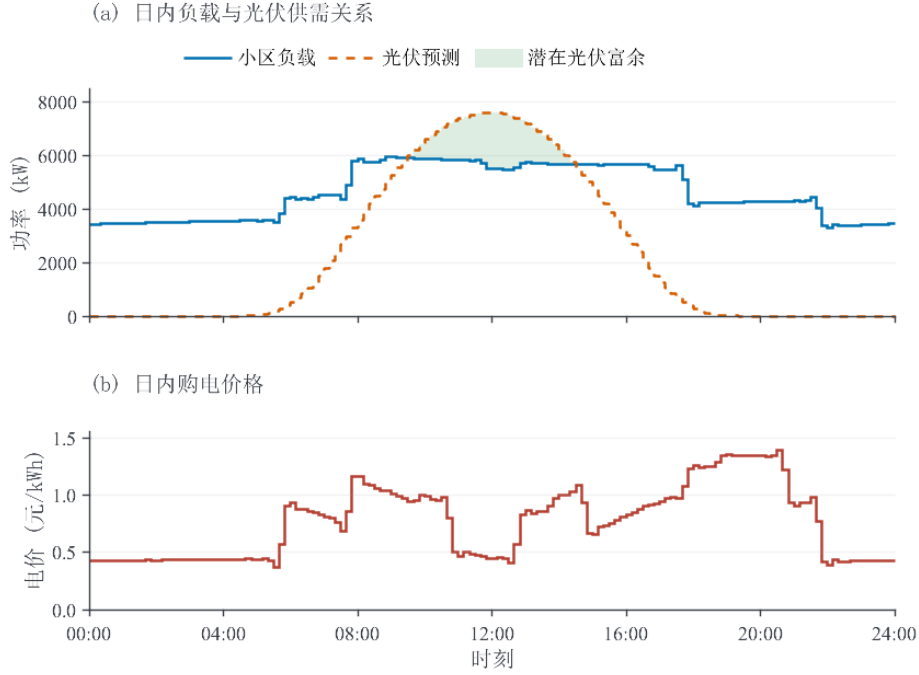
图 2 代表日输入特征：小区负载、光伏预测功率与电价曲线
