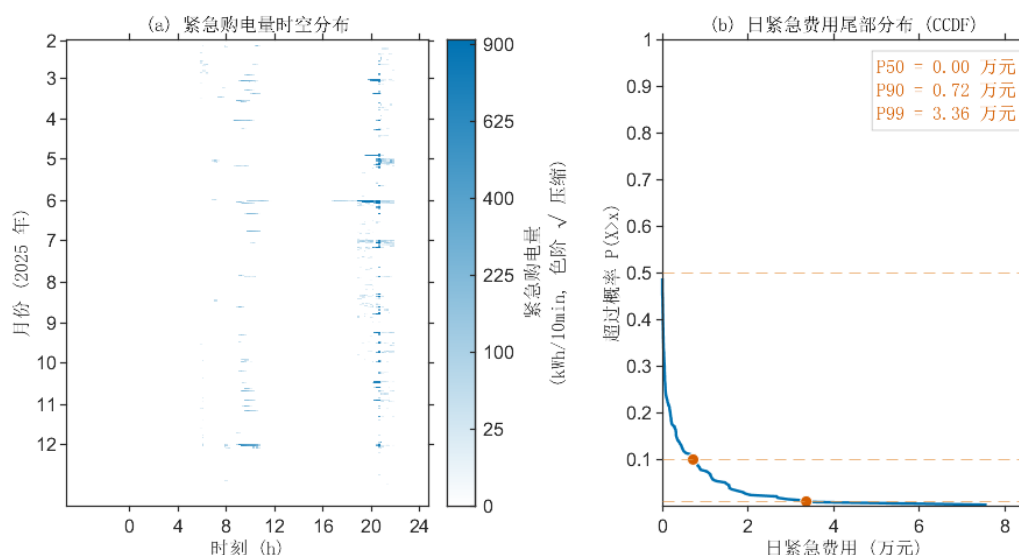
图 10 紧急购电特征：(a) 紧急购电量时空分布；(b) 日紧急购电费用分布
