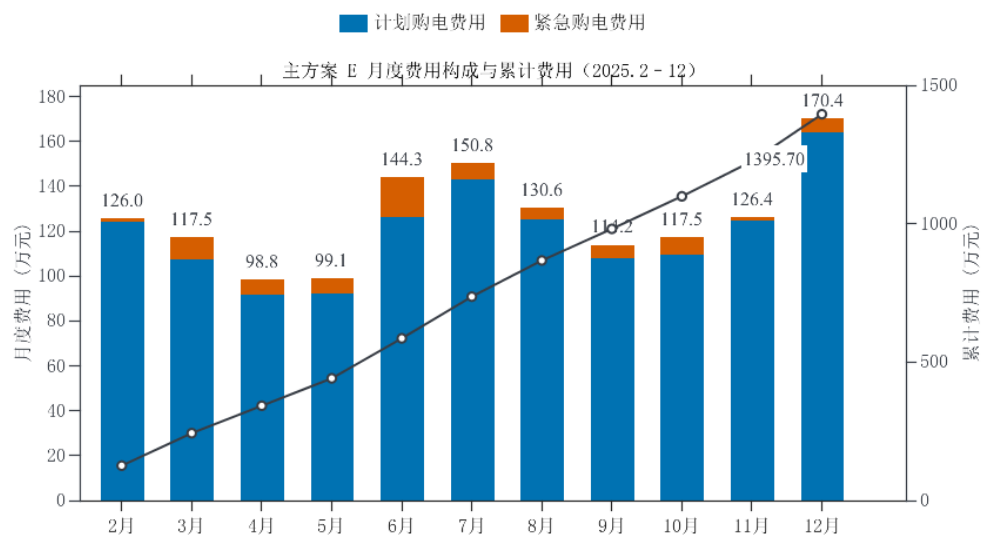
图 9 月度费用构成与累计费用
