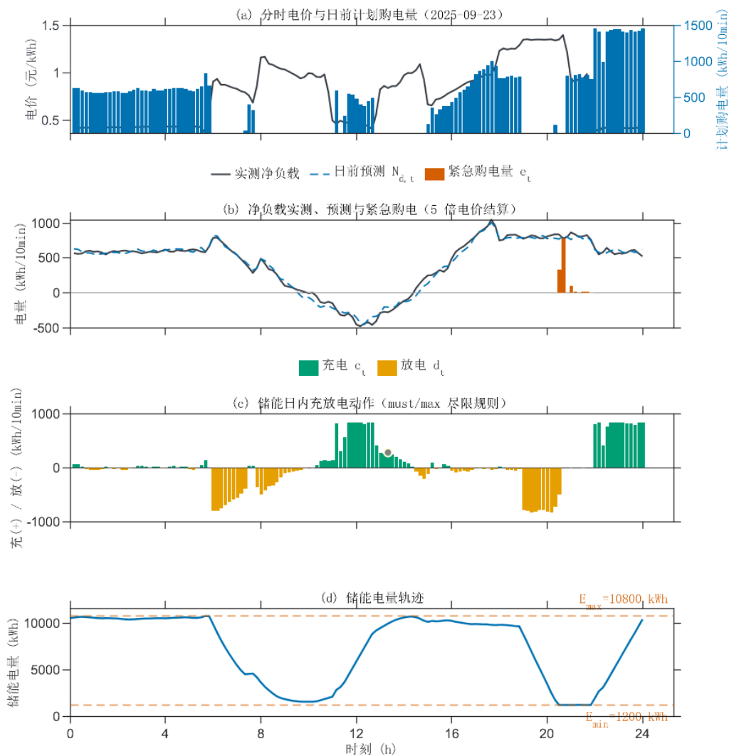
图 7 指定日期的调度细节：(a) 分时电价与日前计划购电量；(b) 净负载实测、预测与紧急购电；(c) 储能日内充放电动作；(d) 储能电量轨迹
