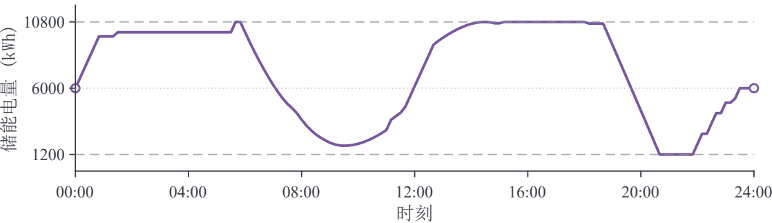
(c) 储能电量与运行边界
