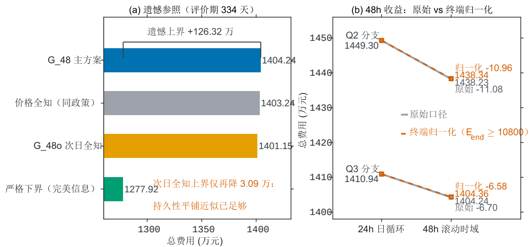
图 20 (a) 各参照方案的横向比较 (万元)：严格下界 1277.92、次日全知上界 1401.15、价格全知 1403.24、主方案 G_48 1404.24、基准 G_fixed 1410.94、基准 F_fixed 1449.30、主方案 F_48 1438.23；(b) 年末终端归一化前后的对照，48 小时时域版的收益在共同终端条件下保持 (1438.34 对 1449.30、1404.36 对 1410.94)
