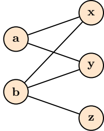
Grafo G_2
