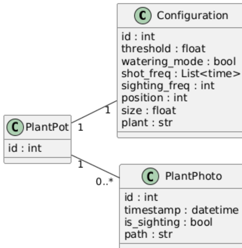
Figura 5: Diagramma del modello di dominio e delle entità principali.
