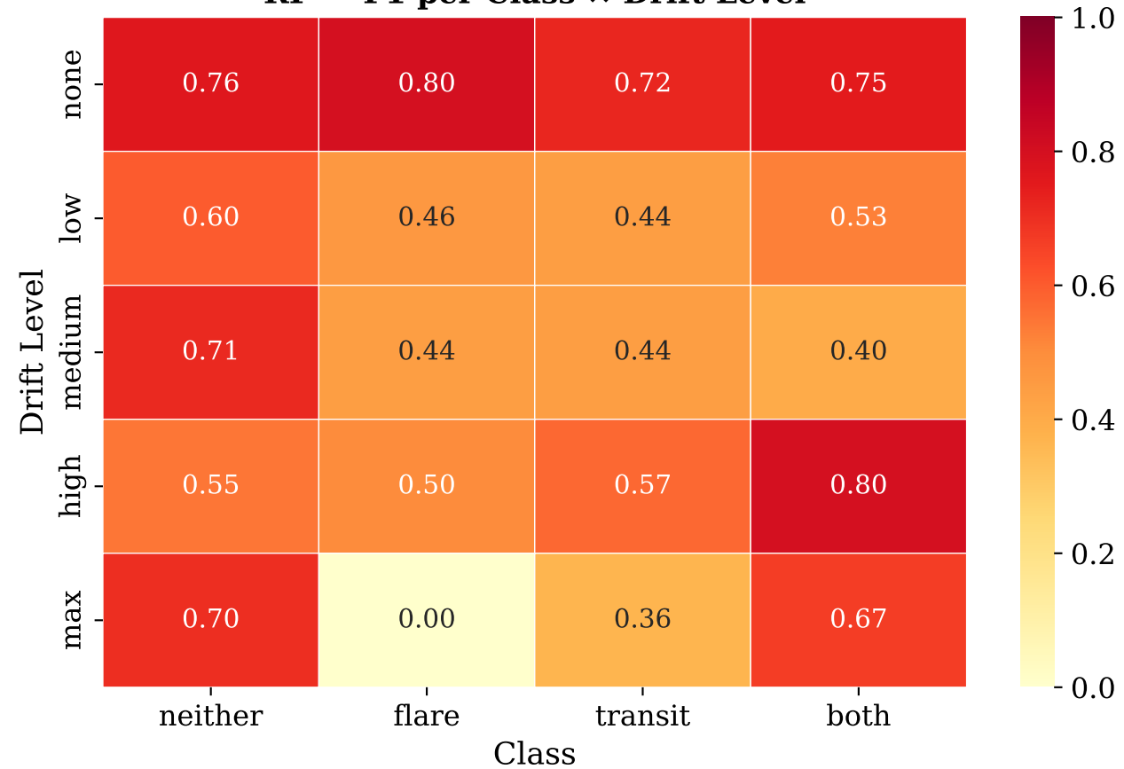
RF — F1 per Class × Drift Level
