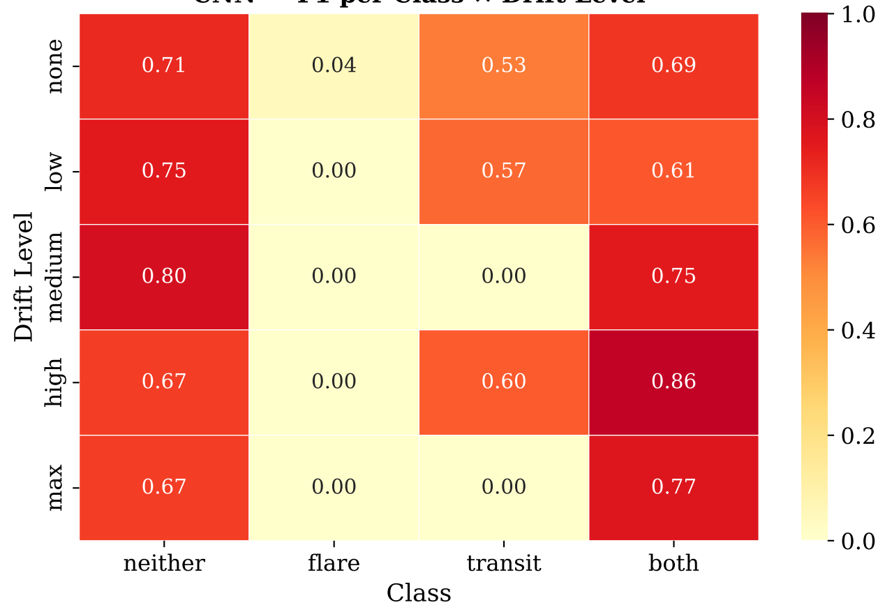
CNN — F1 per Class × Drift Level
