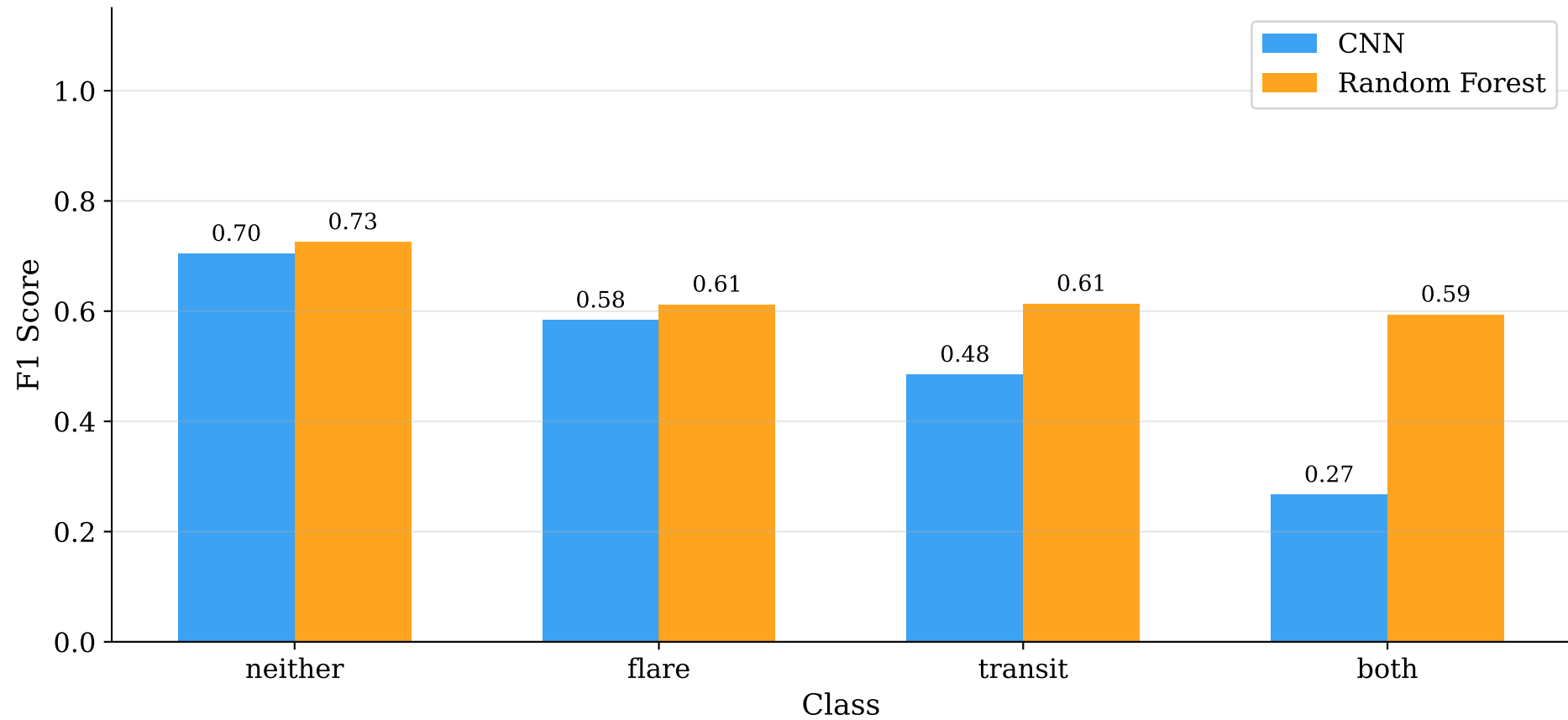
Per-class F1 Score — CNN vs. Random Forest
