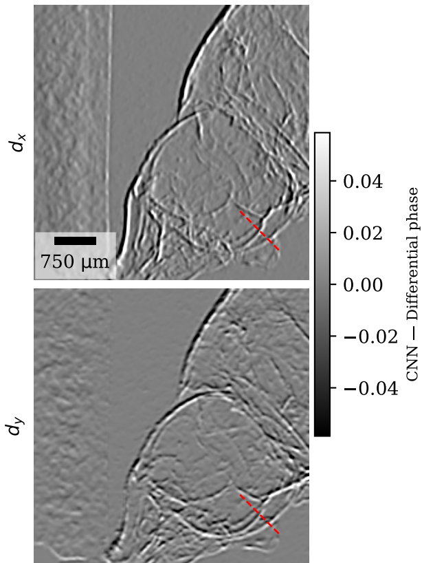
CNN
