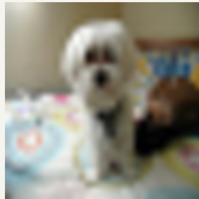
224 × 224 (bicubic)
