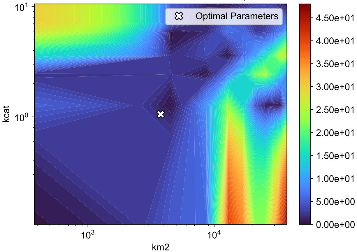
Parameter correlation surface for km2,kcat
