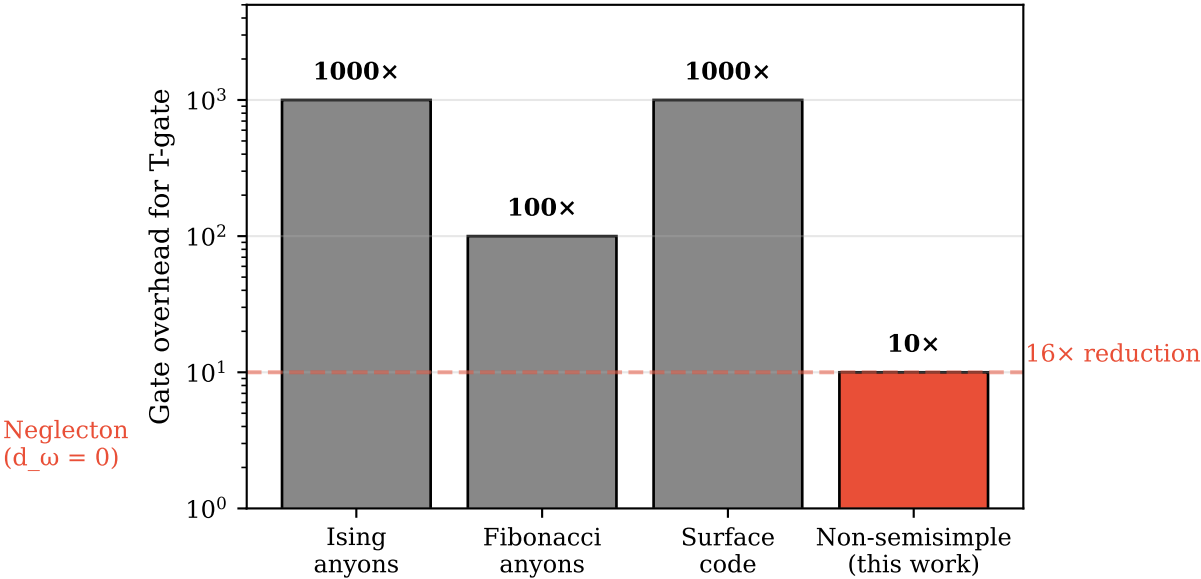
(d) Universality Gate Overhead
